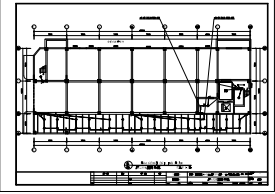
平面布置(照明)
