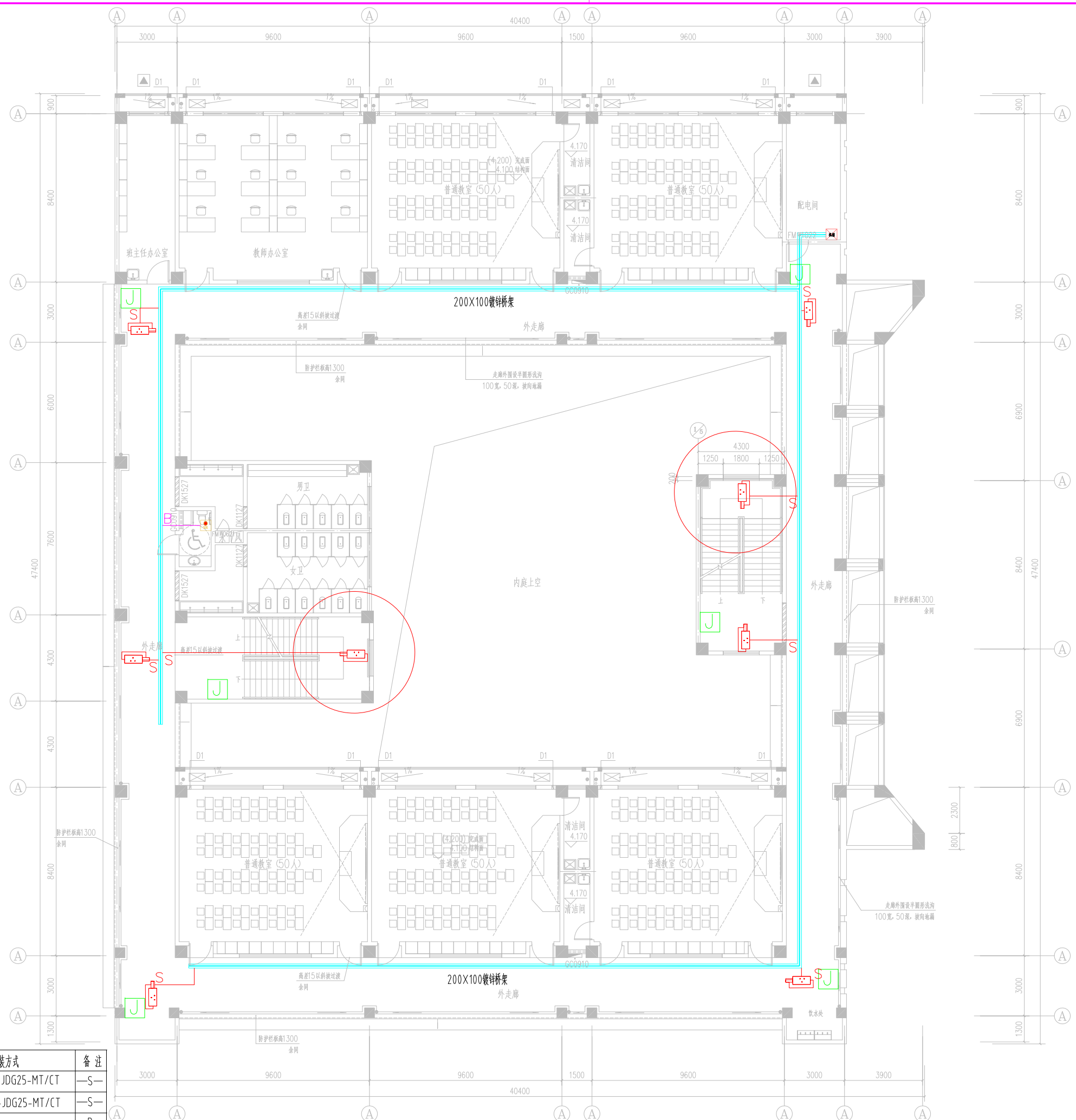
二层平面图 1:100
