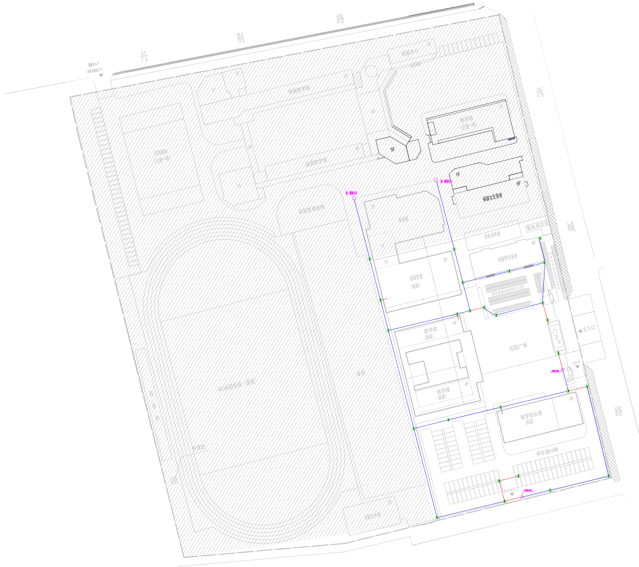
常州市金坛区第四中学改扩建工程室外管路总平面图
