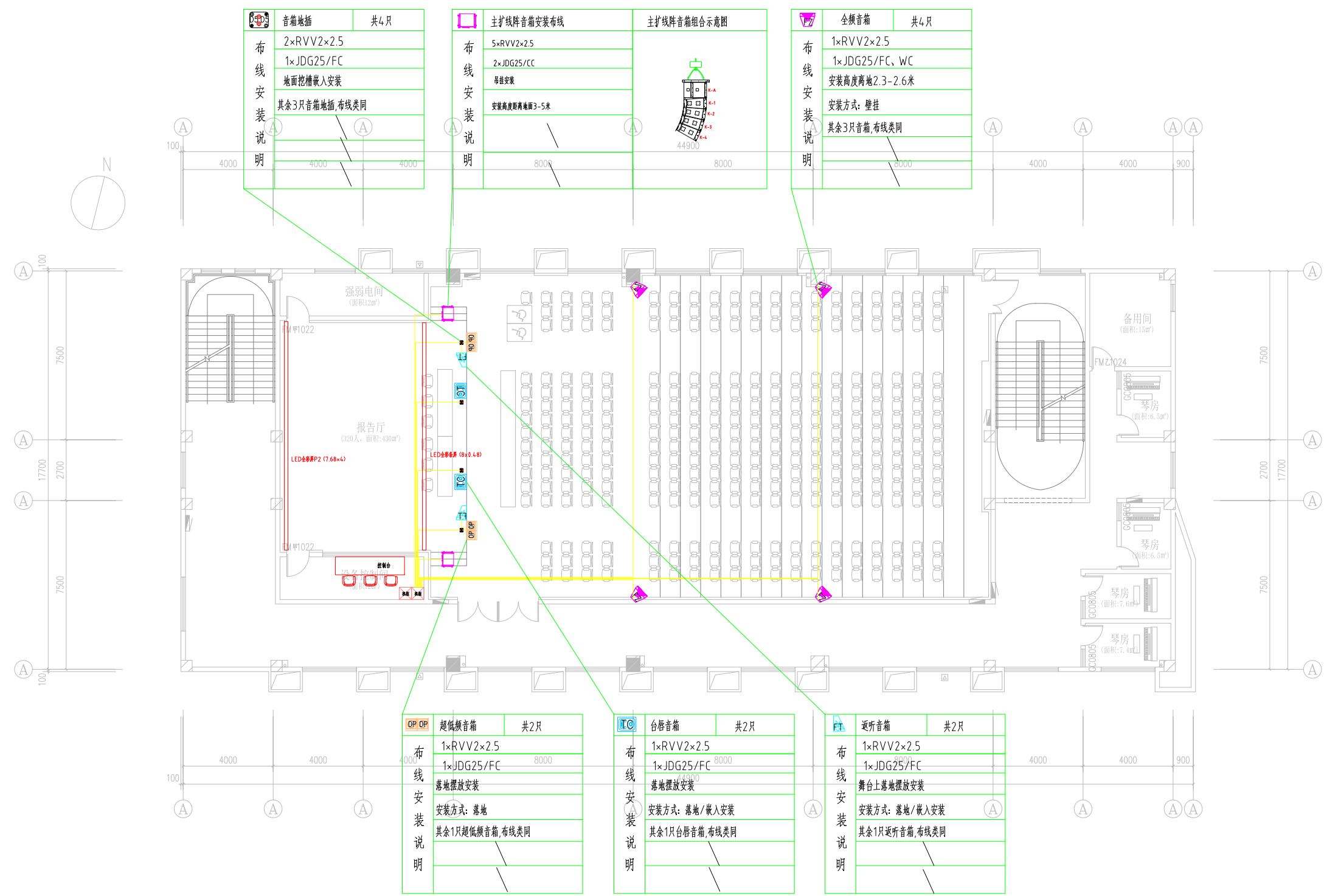
扩声平面布置图 Scale 1:100
