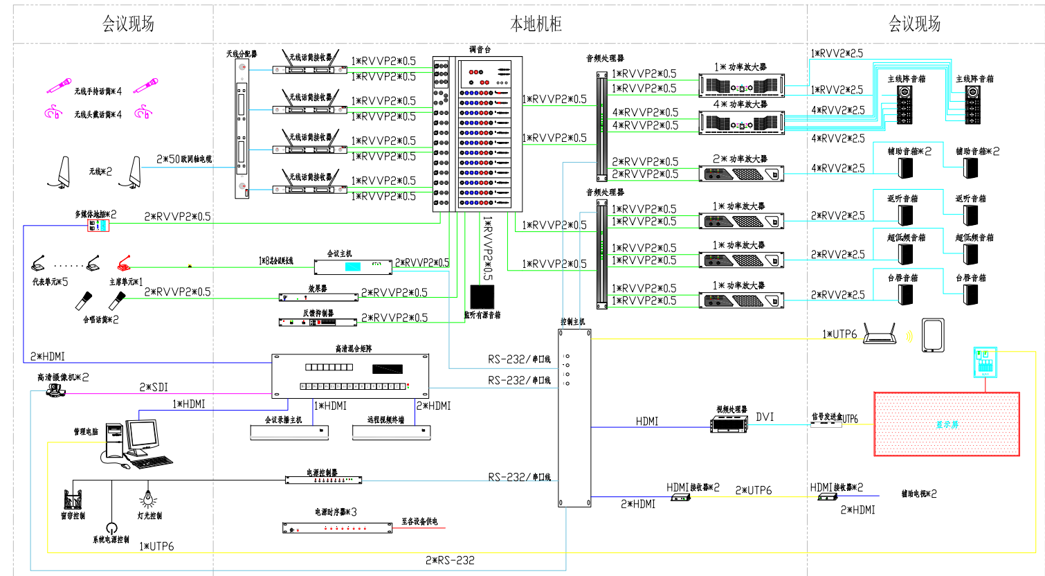
报告厅会议系统图
