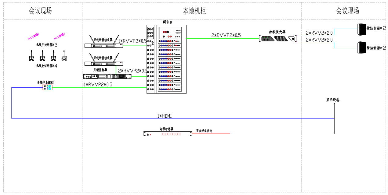
会议室系统图
