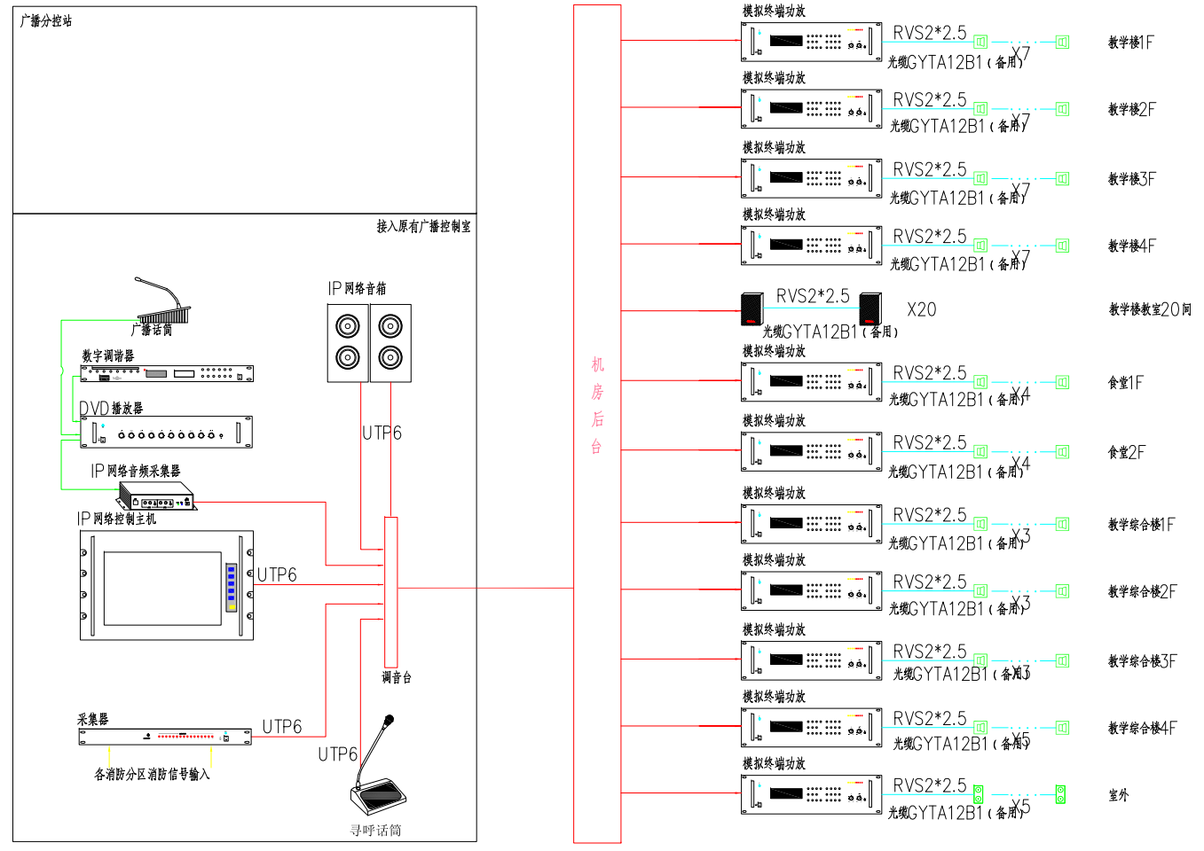
背景音乐系统图
