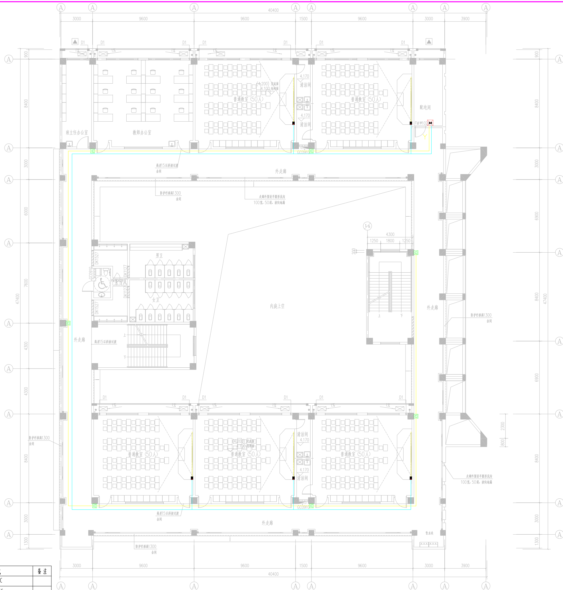
二层平面图 1:100
