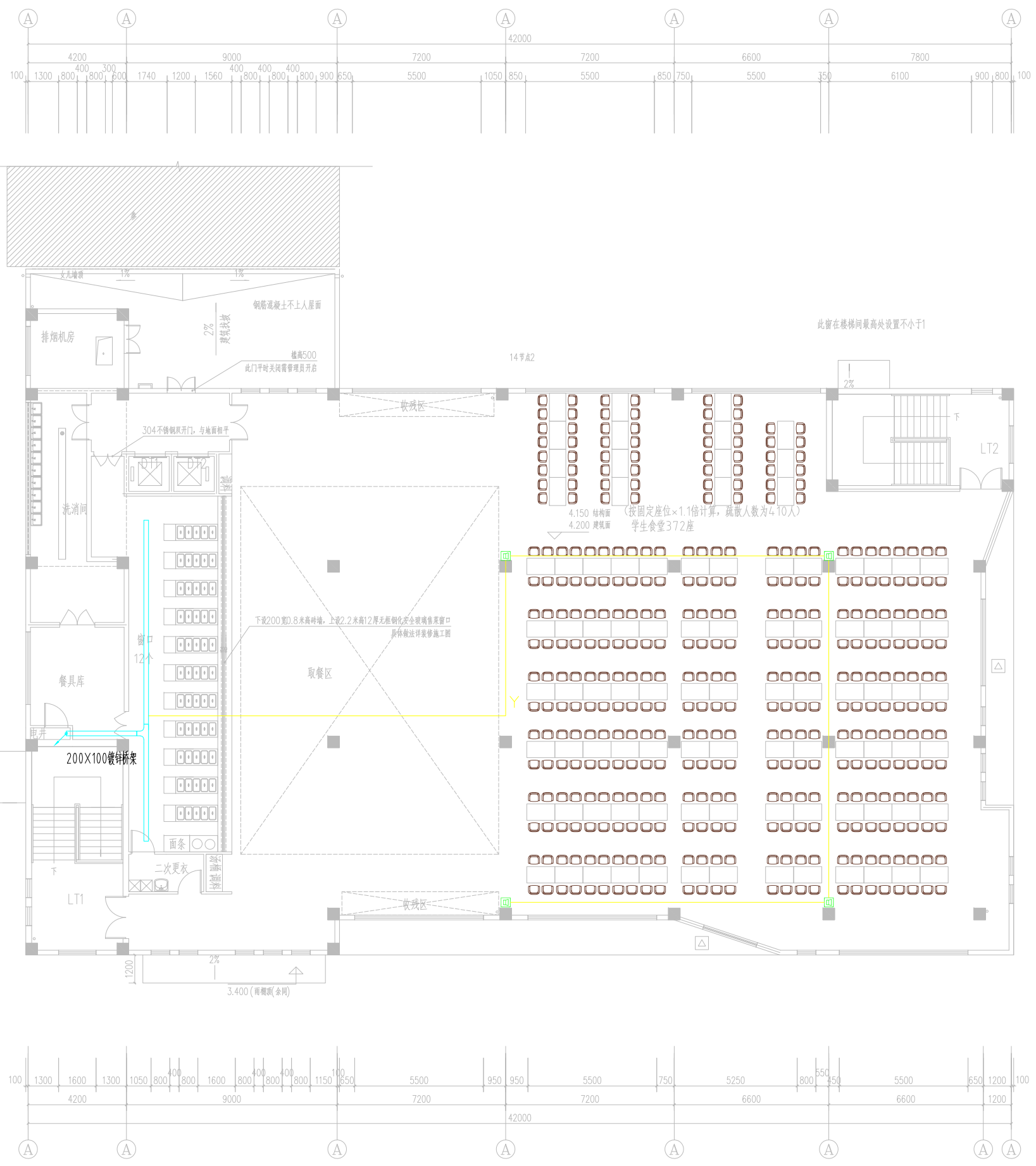
二层平面图 1:100
