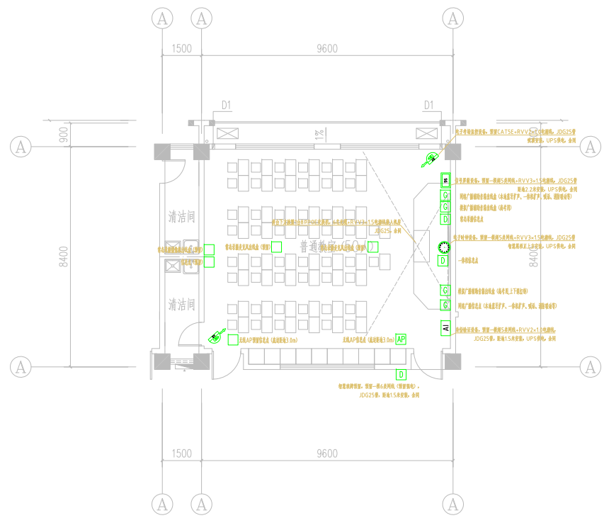
标准化考场 Scale 1:100
