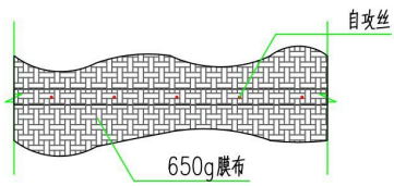
膜布固定节点详图
