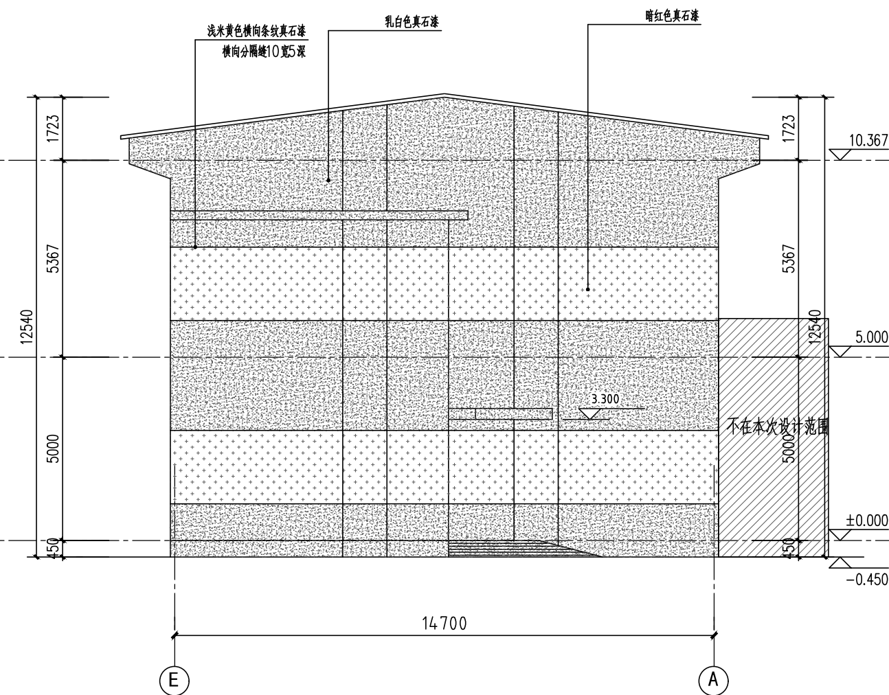
Ⓔ-Ⓐ轴立面 1:100
