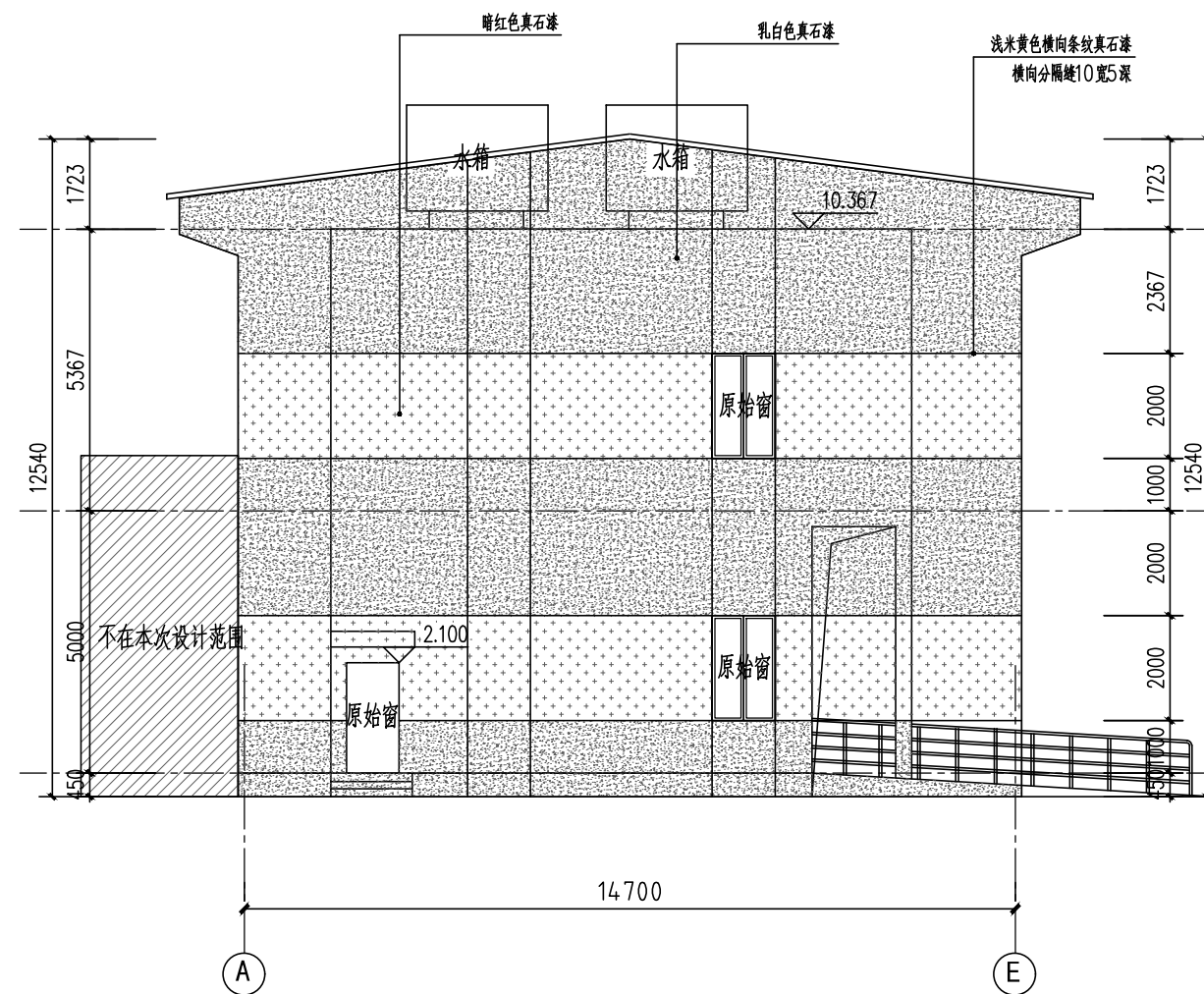
Ⓐ-Ⓔ轴立面 1:100
