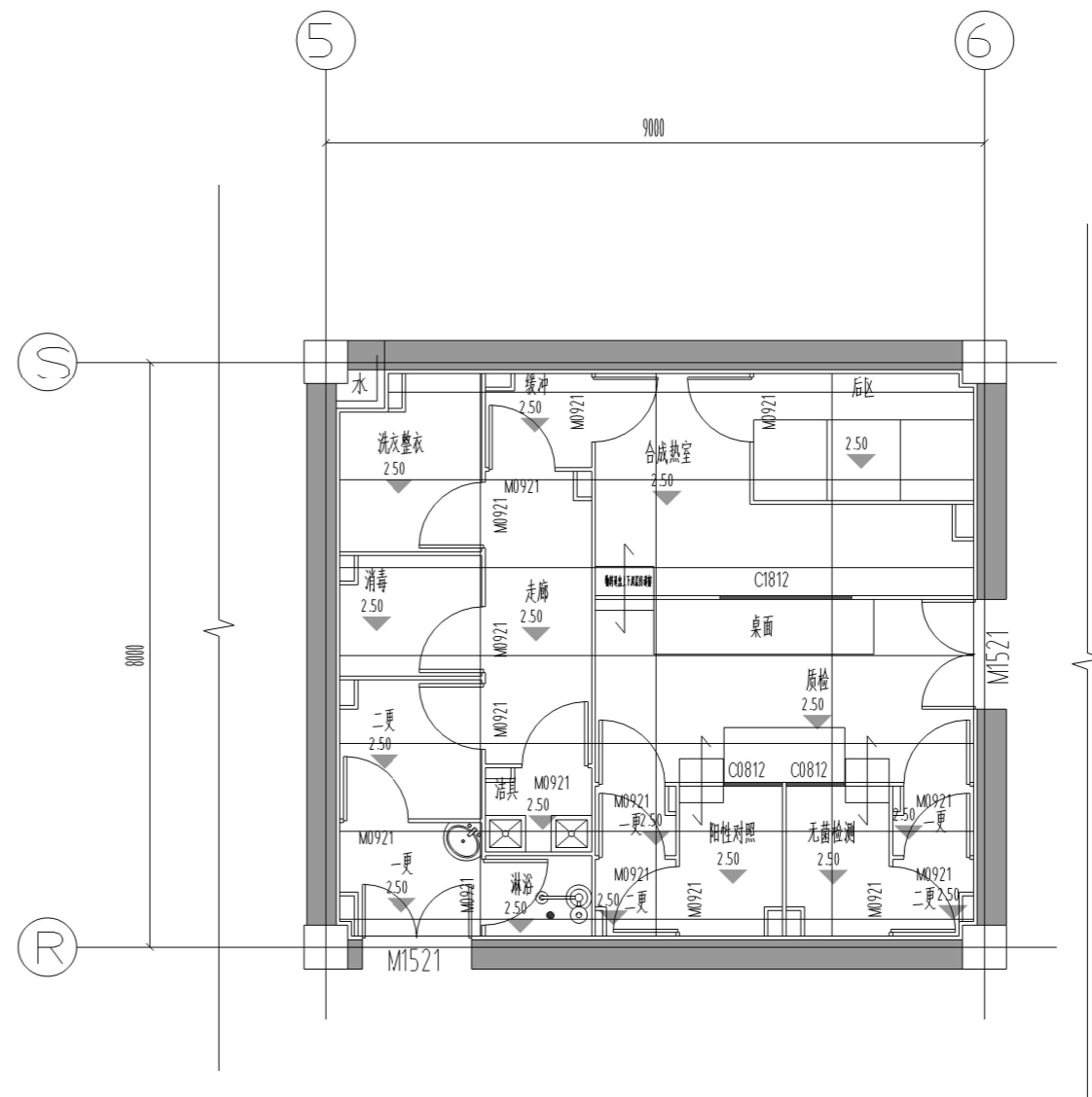
一层吊顶布置图 1:100
