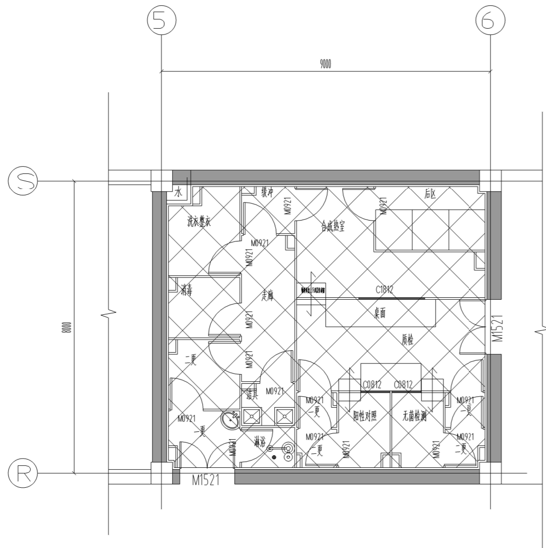
一层地面布置图 1:100
