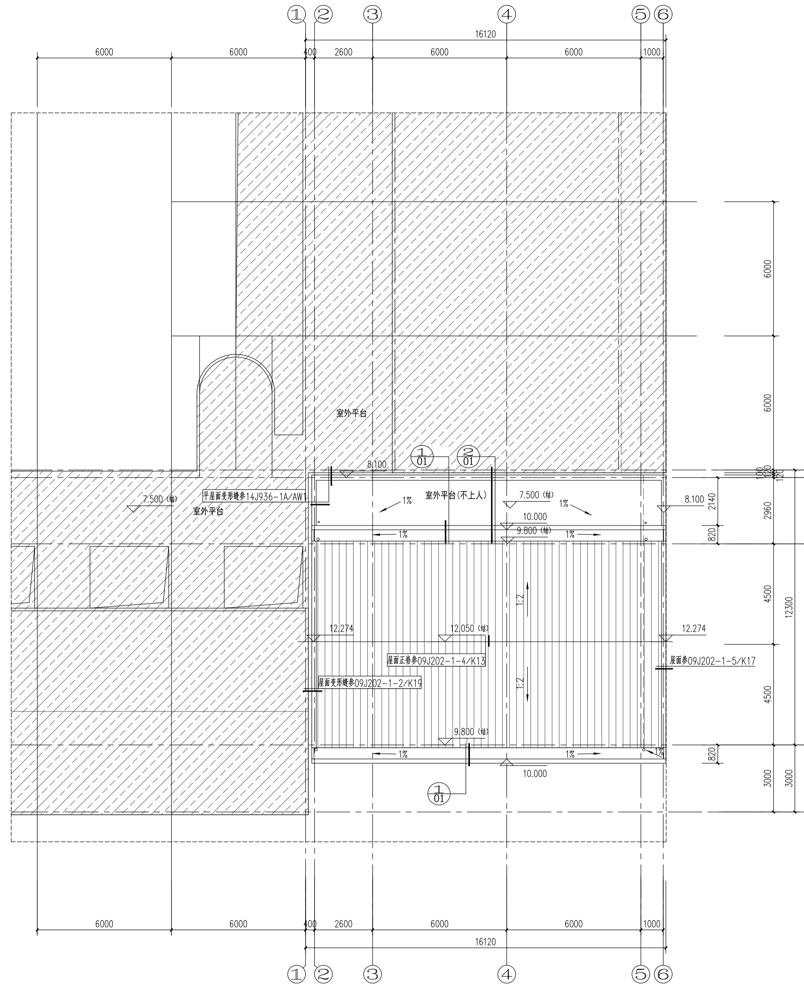
改造后屋顶平面图 1:100
