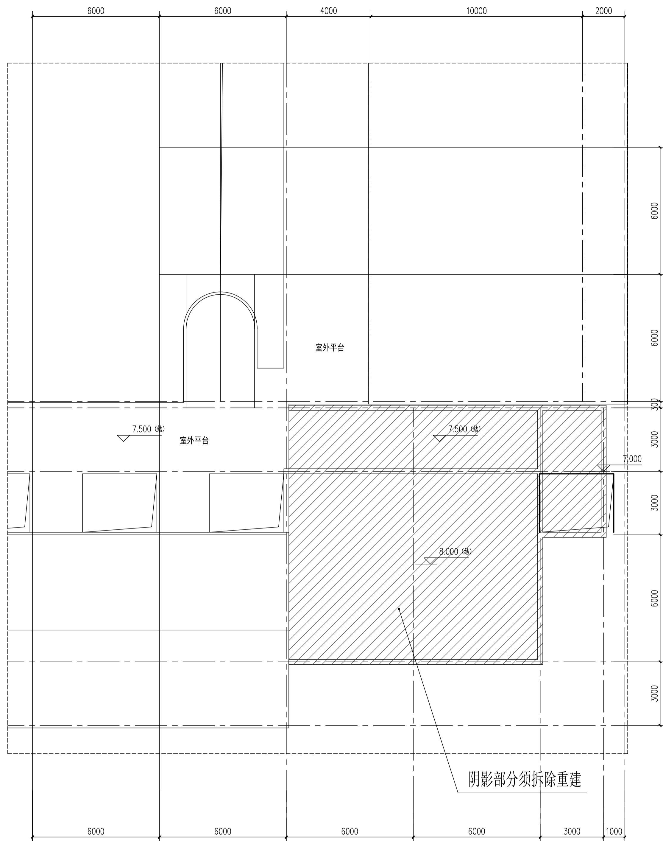
屋顶建筑平面现状图 1:100
