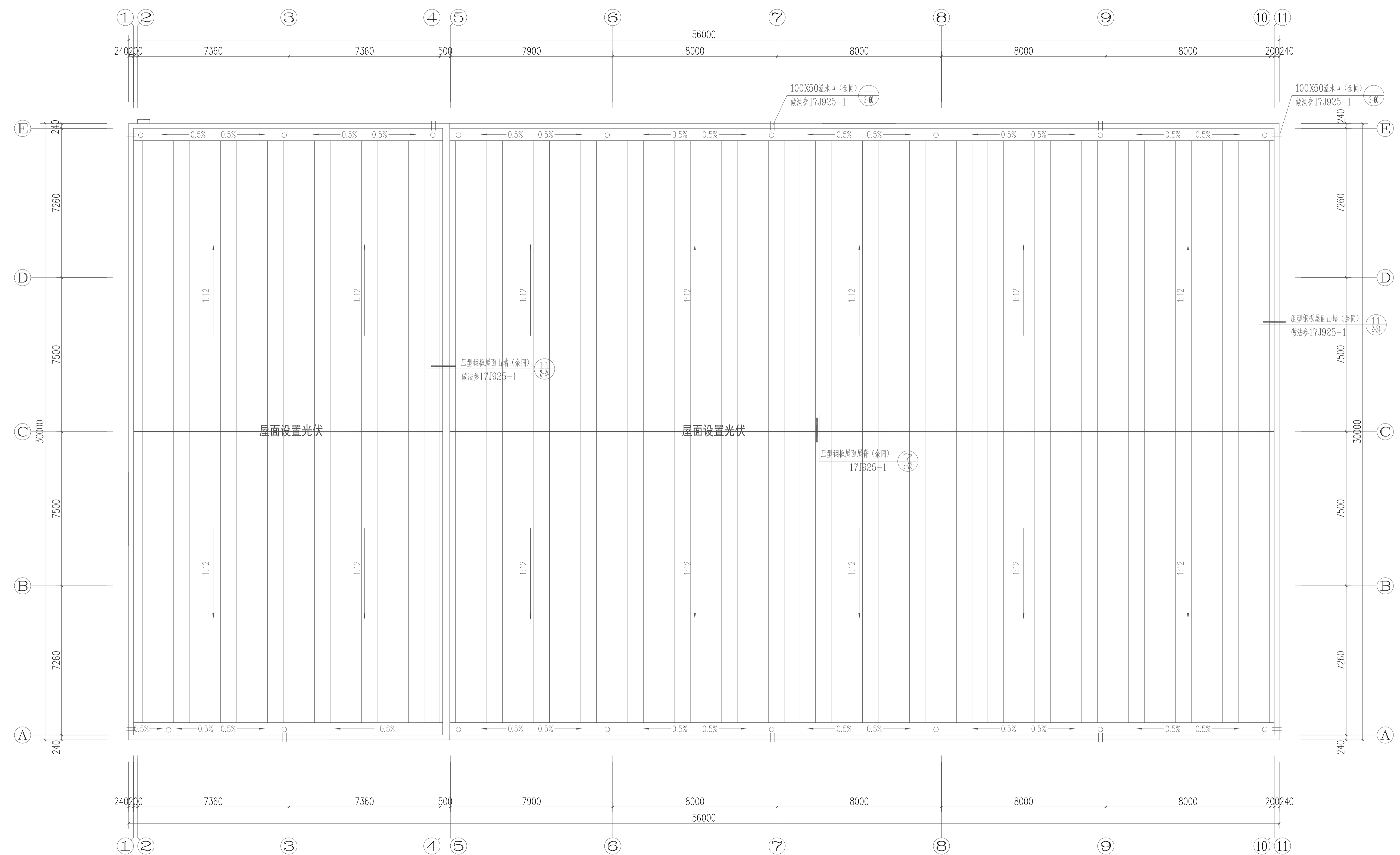
屋面通风平面图 1:100 屋面设置太阳能光伏, 专业厂家二次设计。
