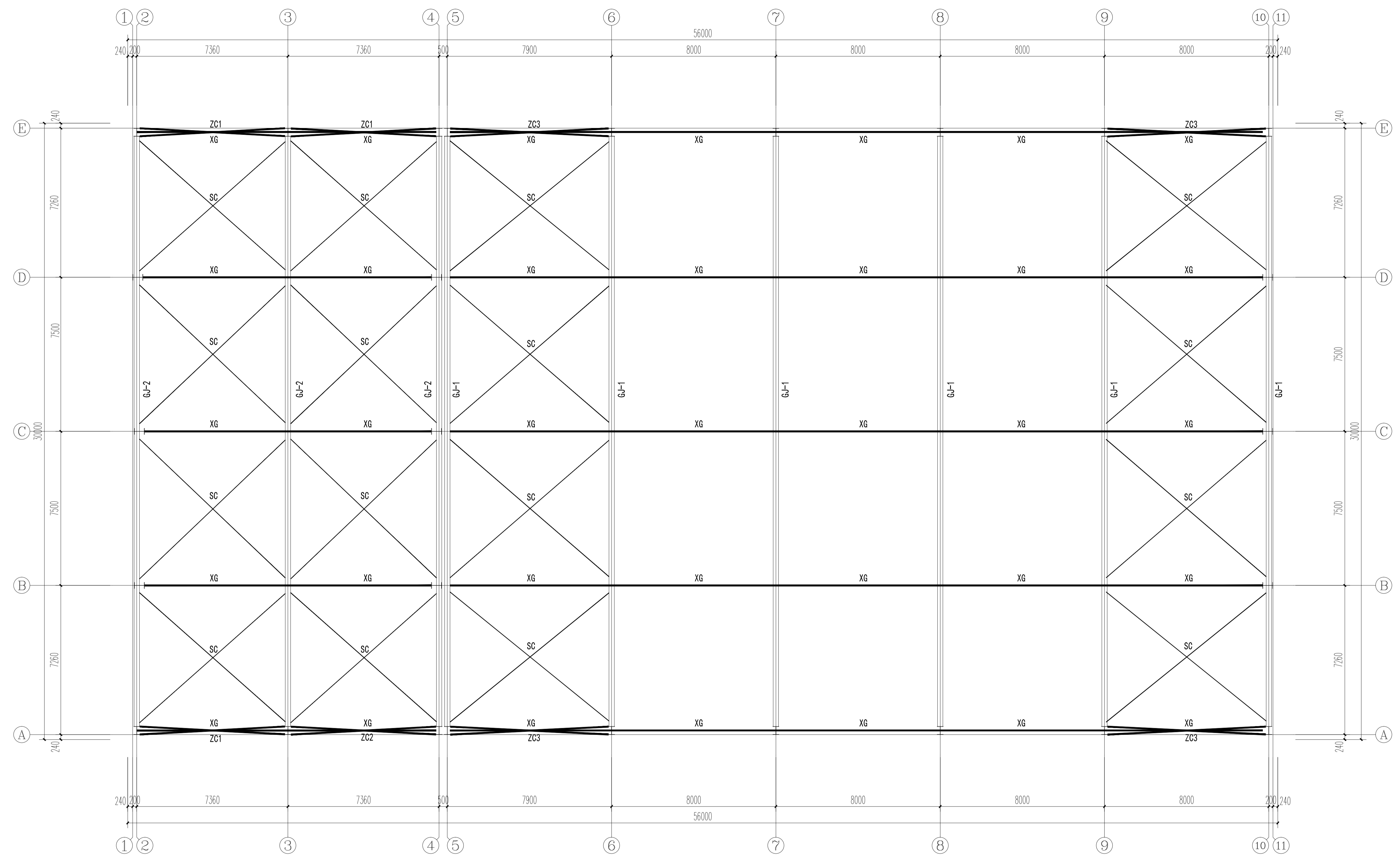
屋面支撑布置图
