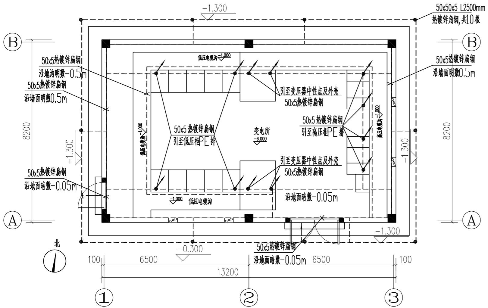
变电所接地平面图 1:100
