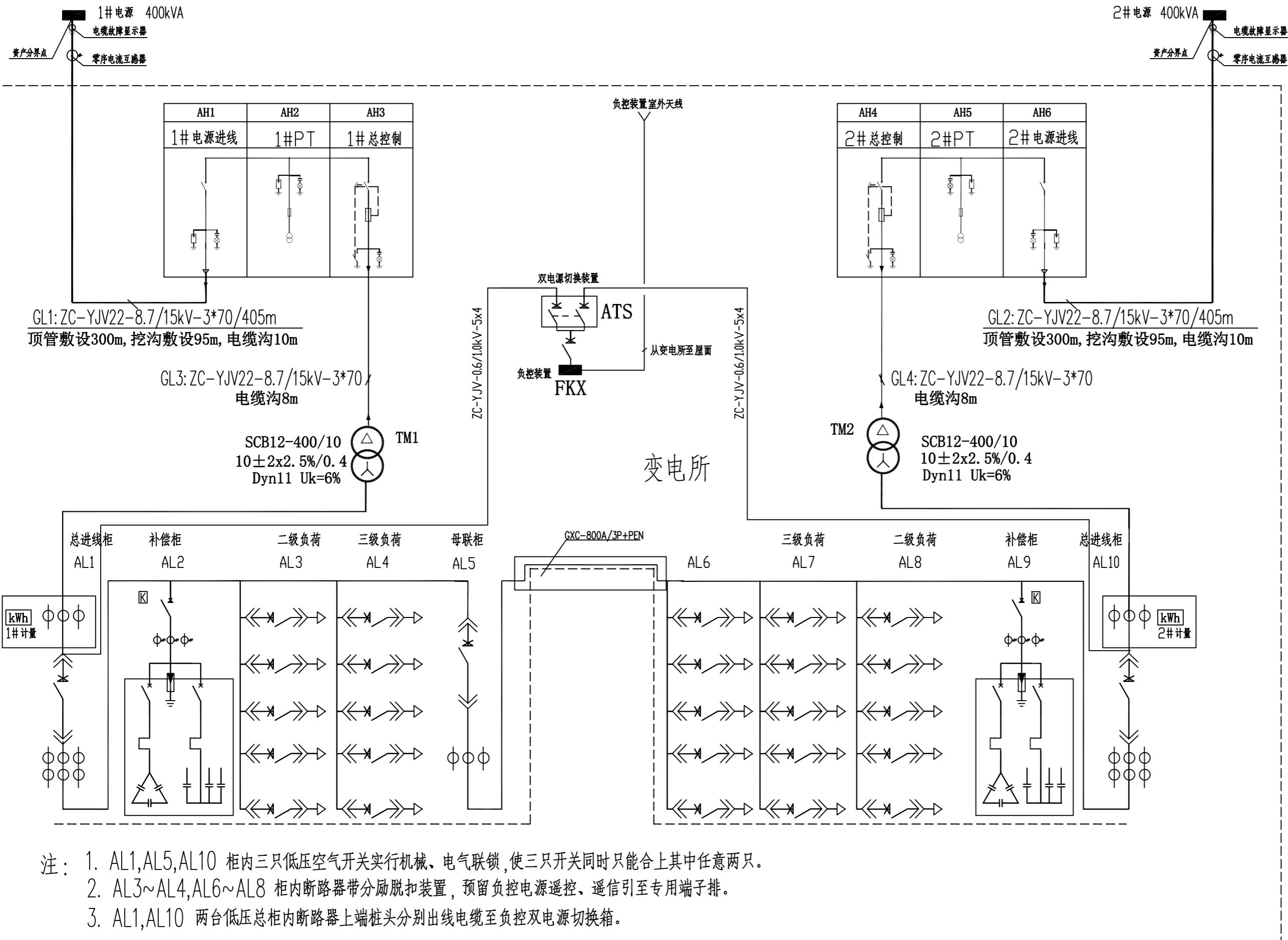
变配电一次接线图 (正视图)
