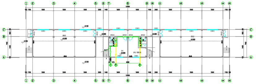
看台一层给排水平面图 1:200
