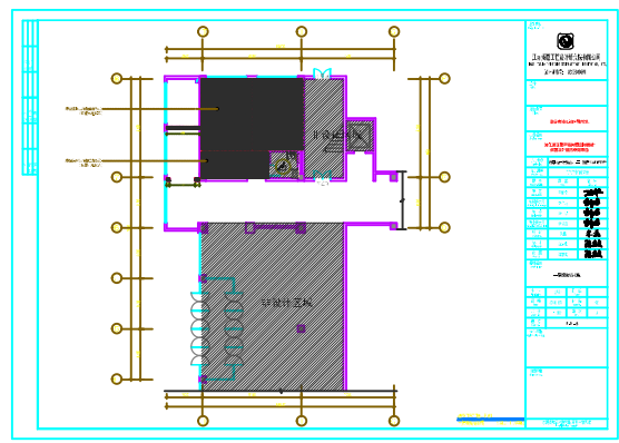
一层原始结构图
