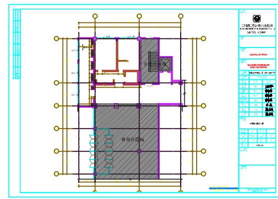
一层完成面尺寸图
