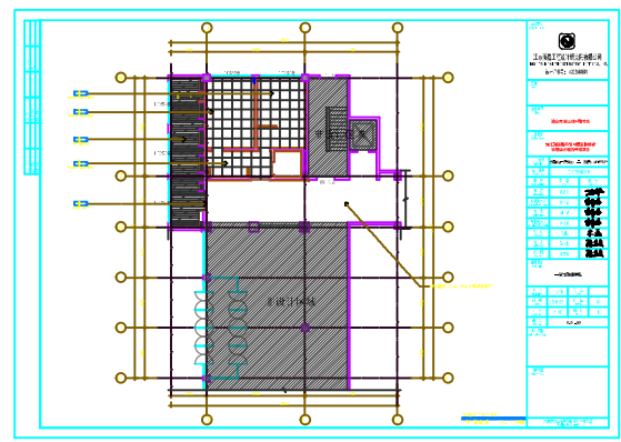
一层地面铺装图
