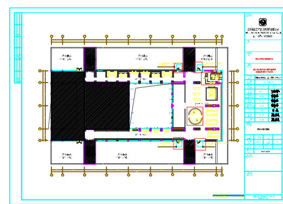
四层平面布置图
