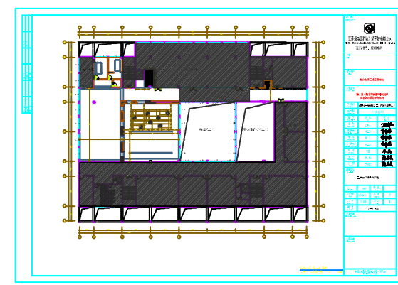
二层天花造型尺寸图
