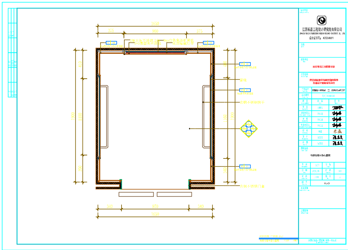
电梯桥箱平面布置图
