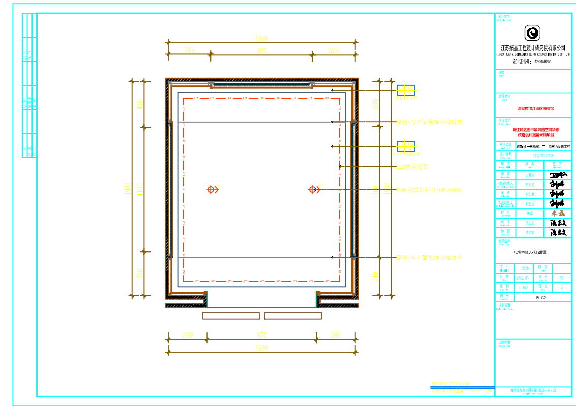
电梯桥箱天花布置图
