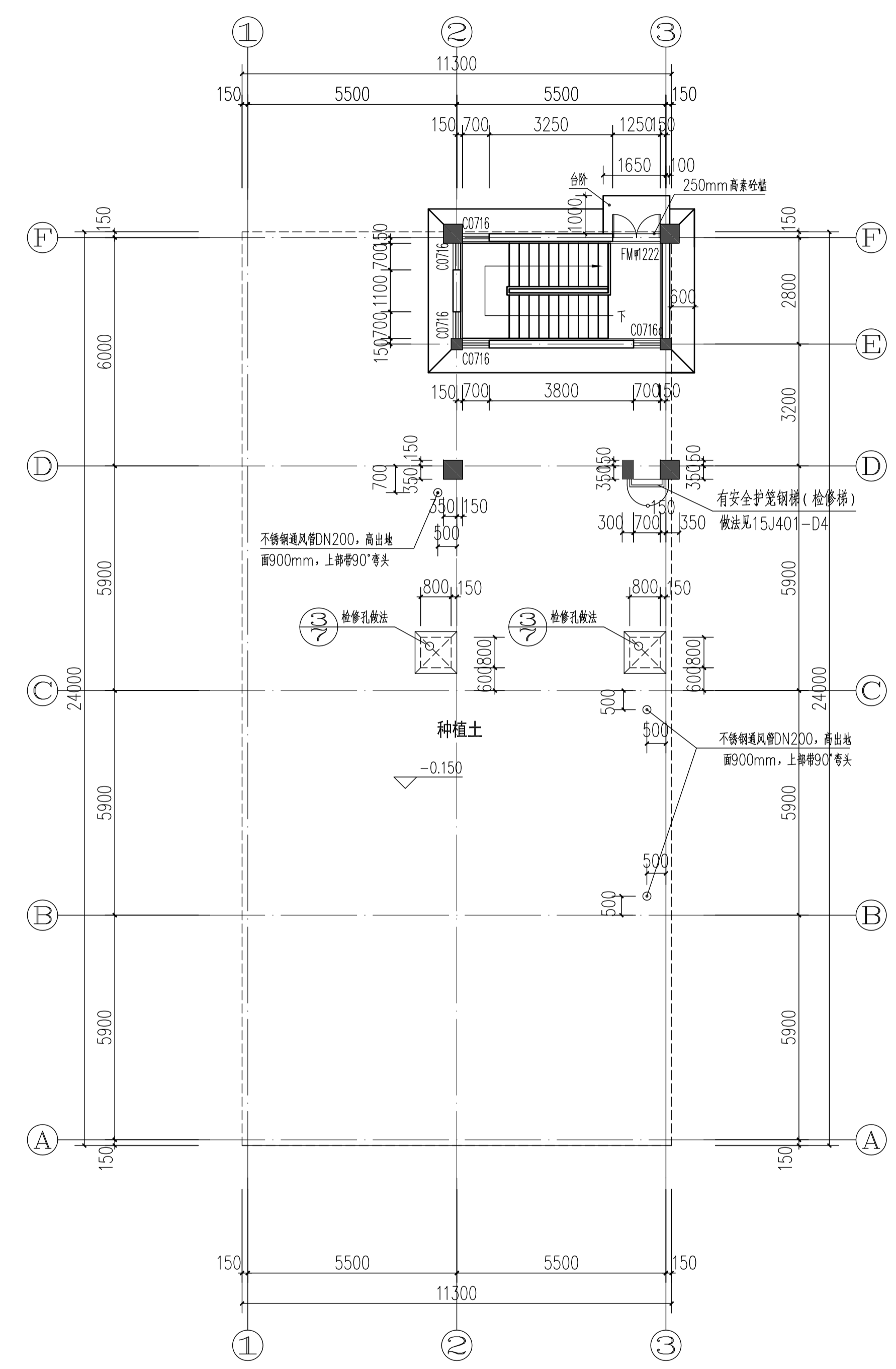
地上层平面图 1:100 本层建筑面积: 17.53m²
