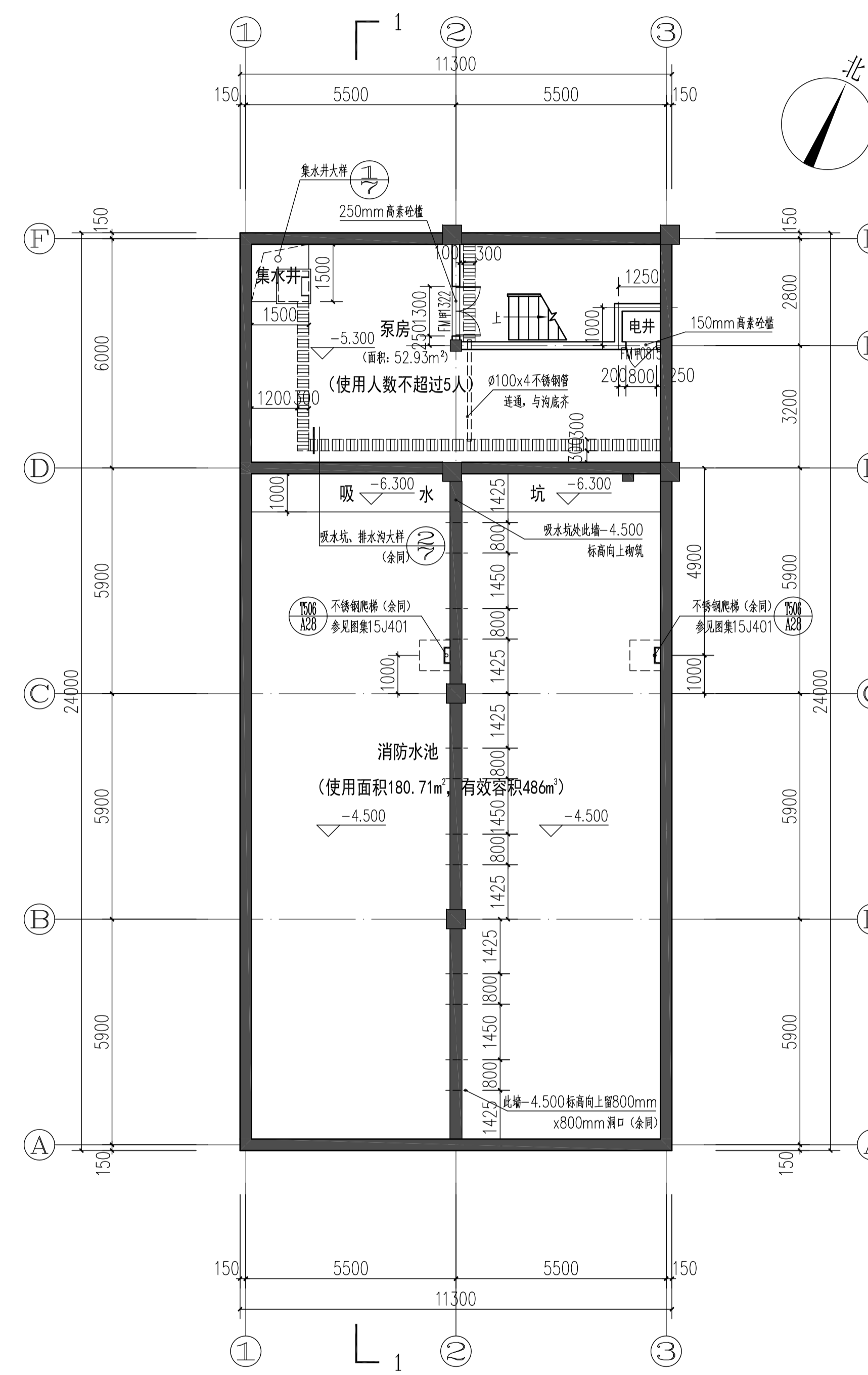
地下层平面图 1:100 本层建筑面积(不计容): 271.56m² 总建筑面积: 289.09m²
