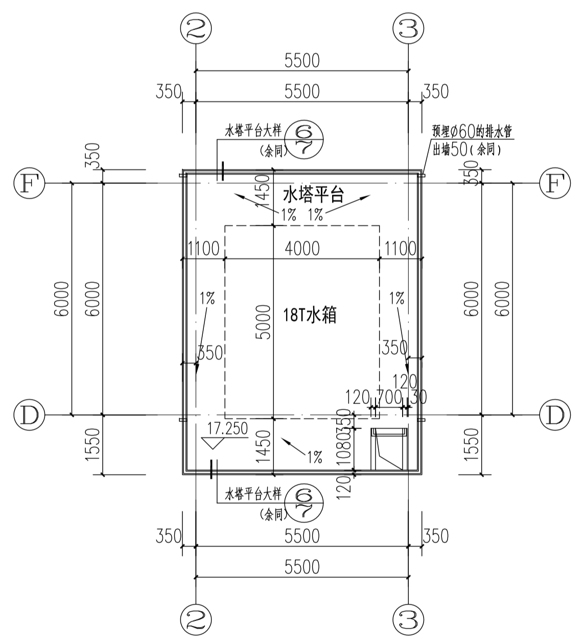
标高17.250处平面图 1:100
