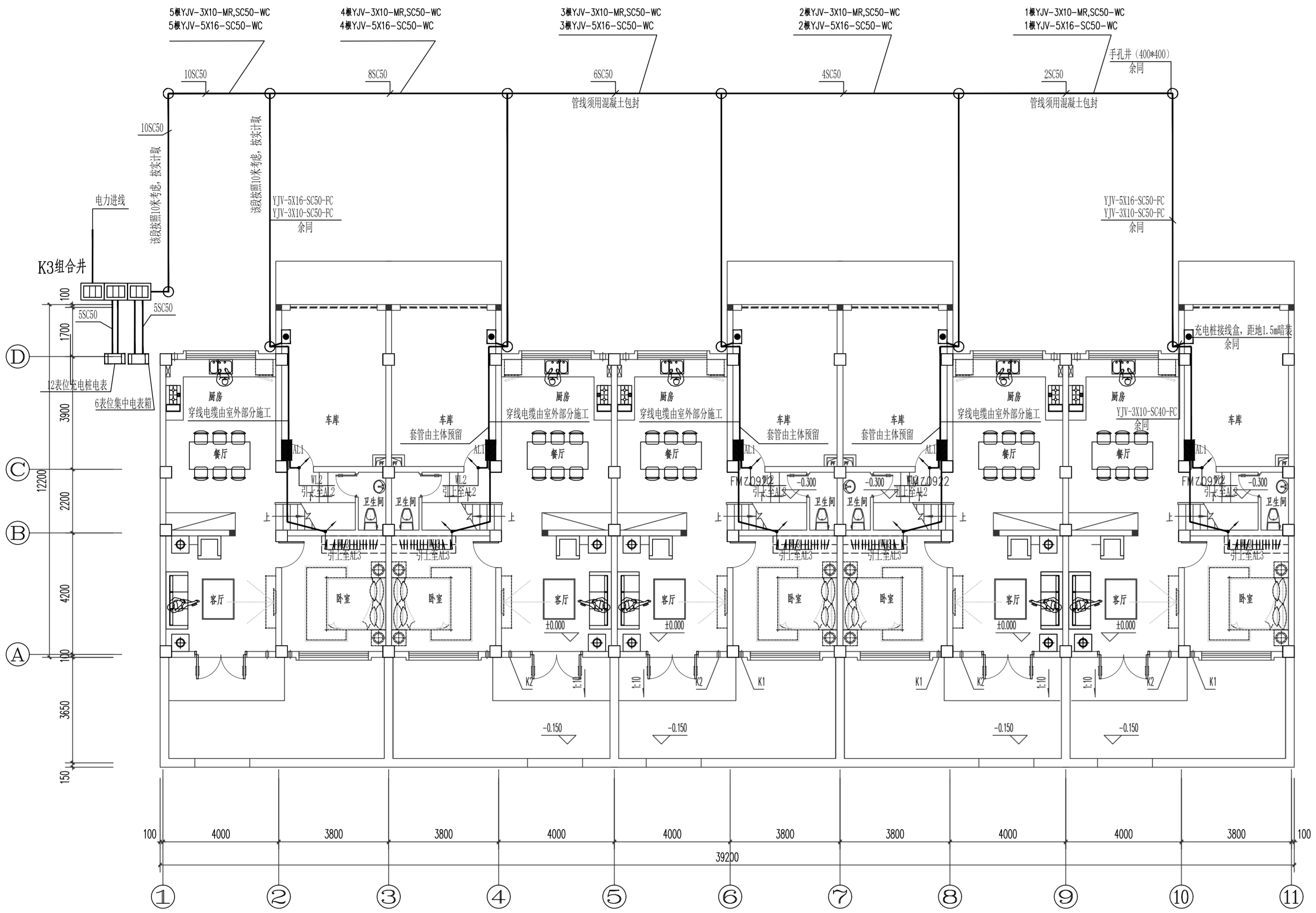
2#楼一层配电网平面图 1:100
