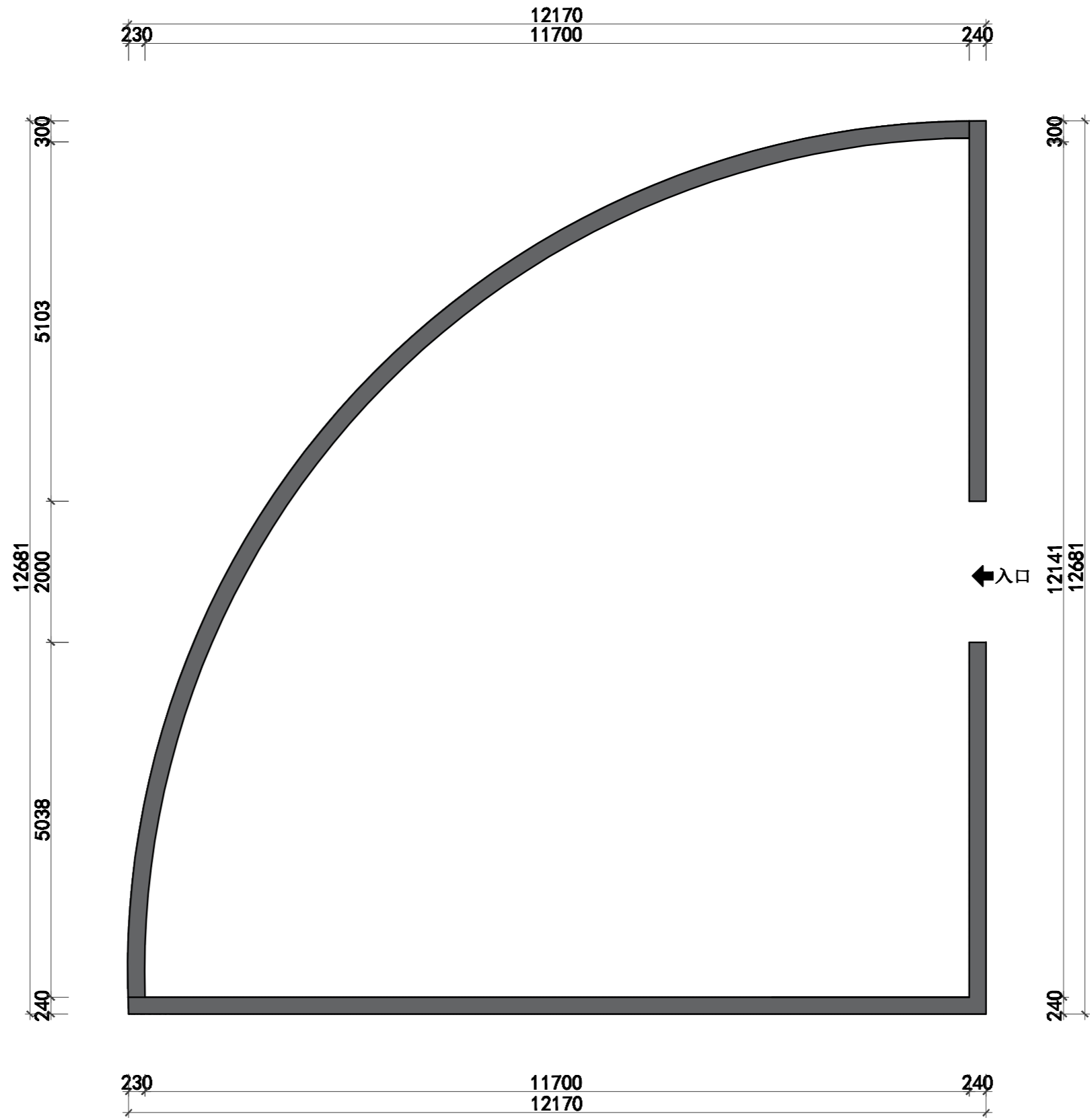
孙园派出所党建阵地原始结构图
